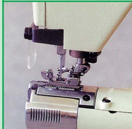
调节式布诱导器、活动压脚舌。 Regulating fabric guide, adjustable guide of presser foot.
